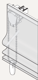
Manœuvre chaînette relevage lacette
